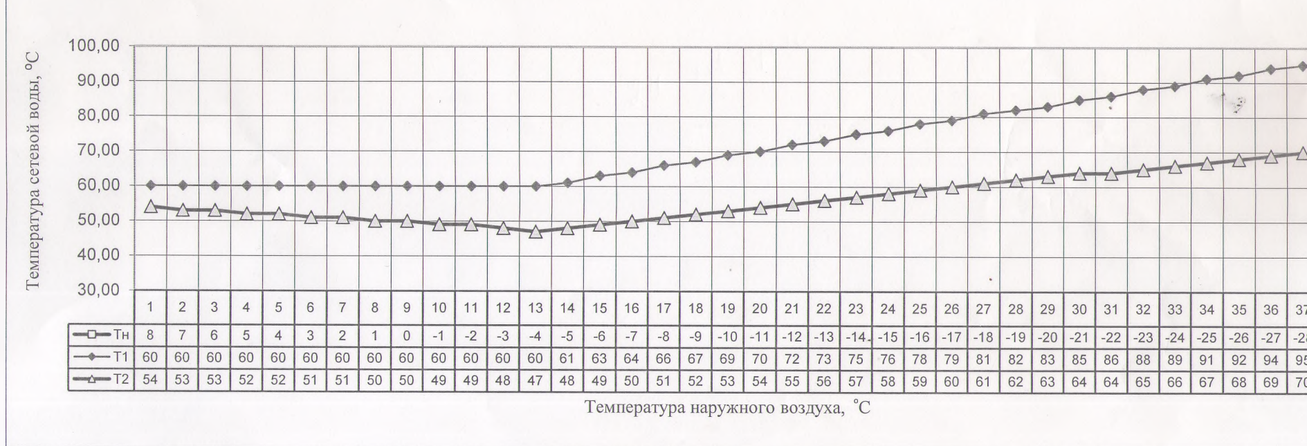
Температурный график регулирования отпуска тепловой энергии на отопительный сезон 2023-2024 г.г. 95-70 °С для Тимлюйской ТЭЦ
